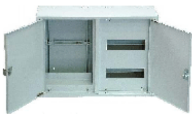
ЩУНЗ-2х9-СИЗ-УХЛ4 Навесной, с цельнометаллическими дверками, под индукционный счётчик до 18 модулей
