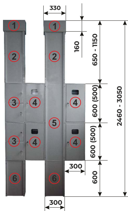
Элементы устройства УЭРМ
