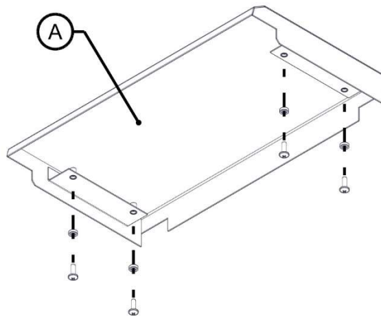
Рис. 1 Козырек защитный шкафов UC2/UC2M.
