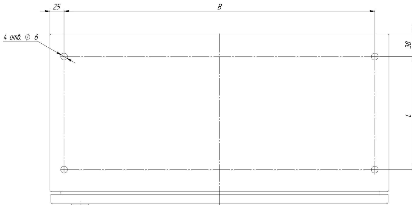
Рис. 2 Шаблон разметки для установки козырька защитного шкафов UC2/UC2M
